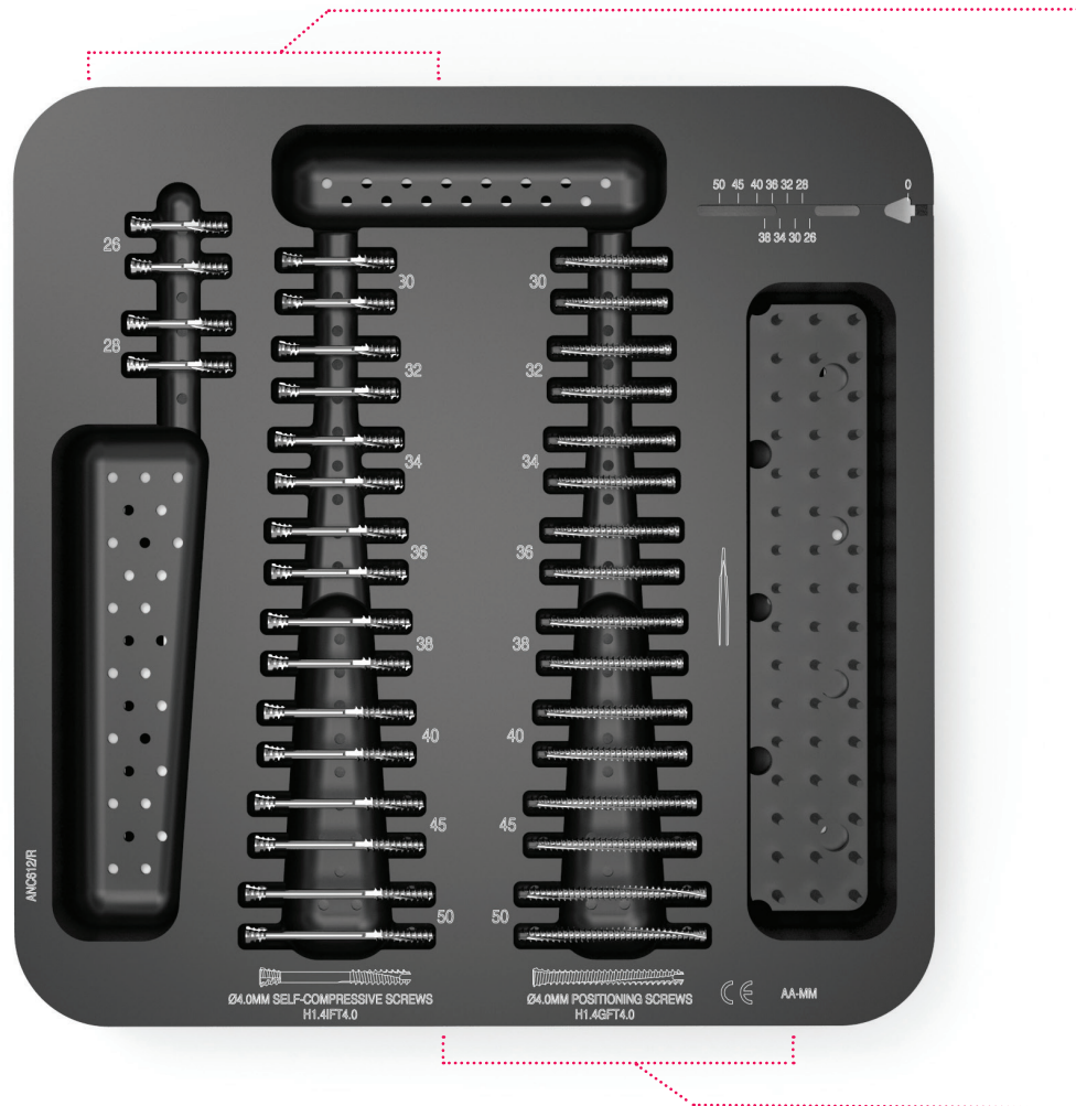
SET - Ø4.0 MM SCREWS DELIVERED NON STERILE (ANC612/B)
